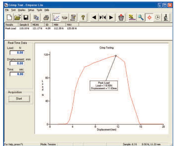
Représentation graphique d'un test (résistance des sertis)
