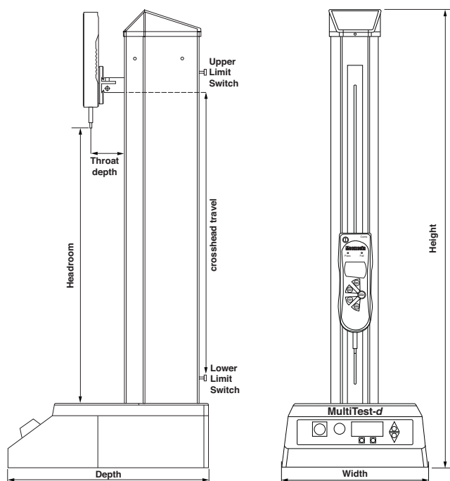
Bancs d'essai présentés avec un instrument de mesure (AFG) fixé sur la traverse.
